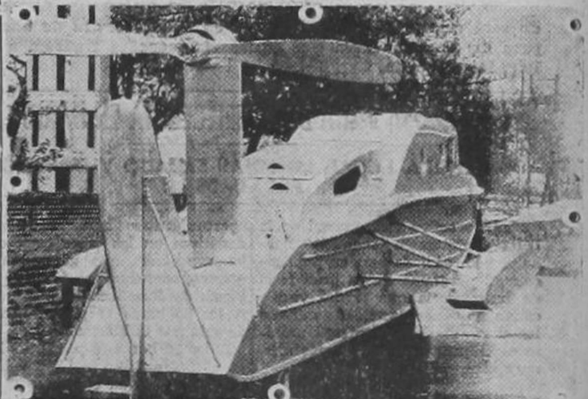
Un nuevo tipo de hidro-gliseur el "Stella-Maris" que se encuentra expuesto actualmente en la Exposición Náutica de París. Lleva un motor marca Morin-Continental de 75 H.P. y alcanzará 55 km. de velocidad a la hora.
